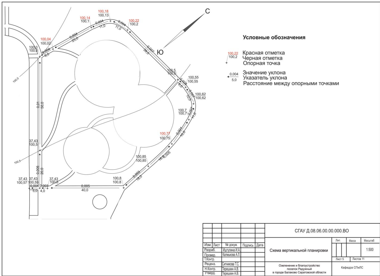
Схема вертикальной планировки в проектных отметках.
