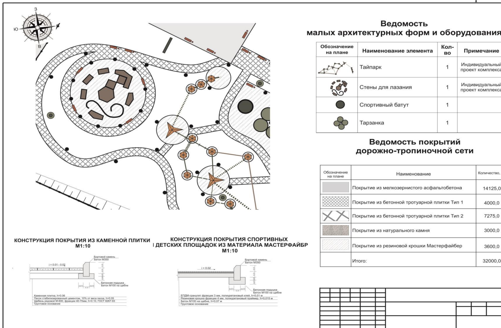
План покрытий дорожно - тропинойной сети и благоустройства территории
