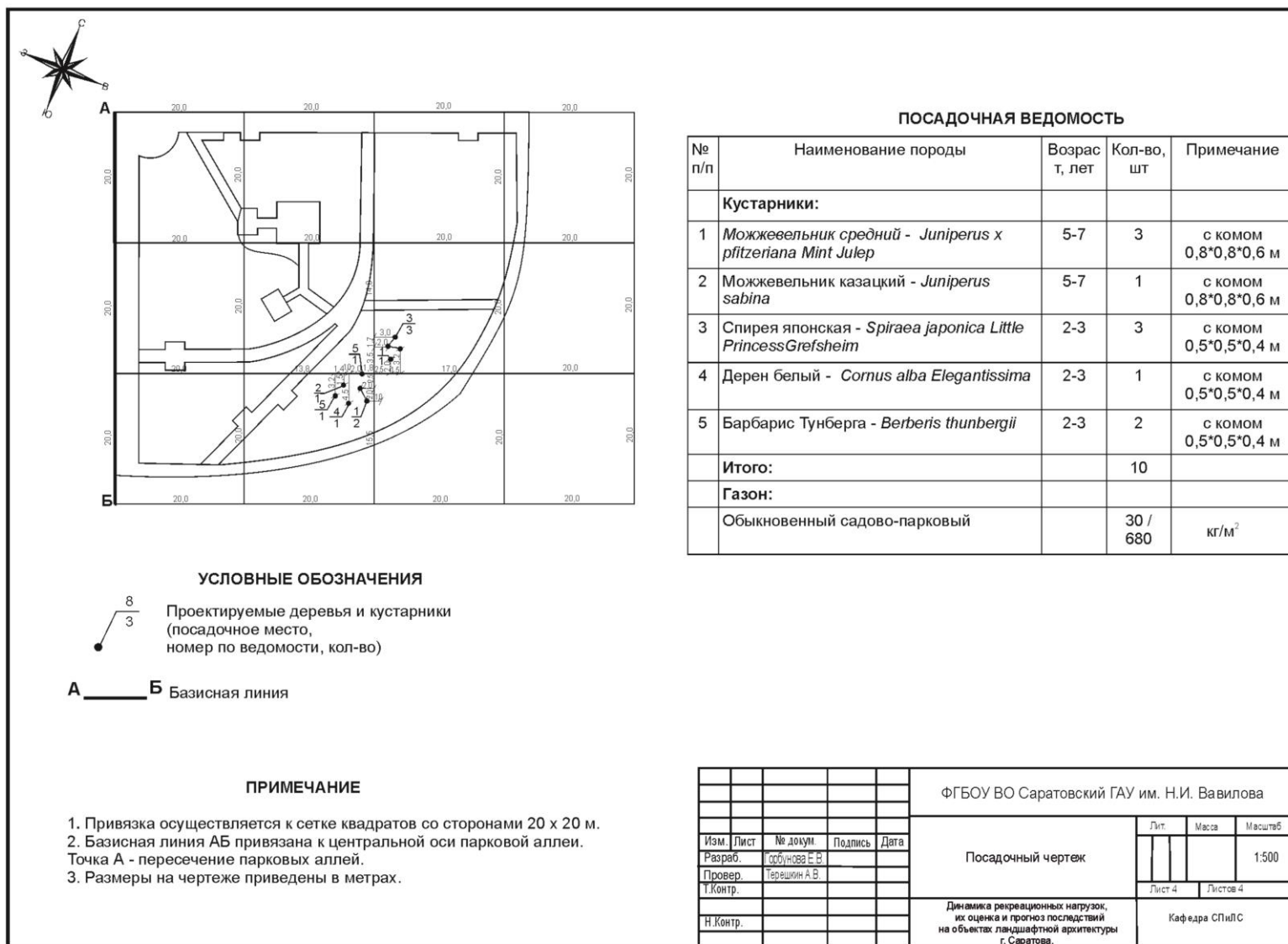
Посадочный чертёж
